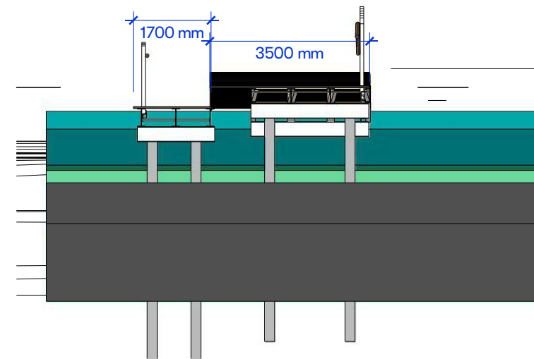
Doorsnede 1:100
