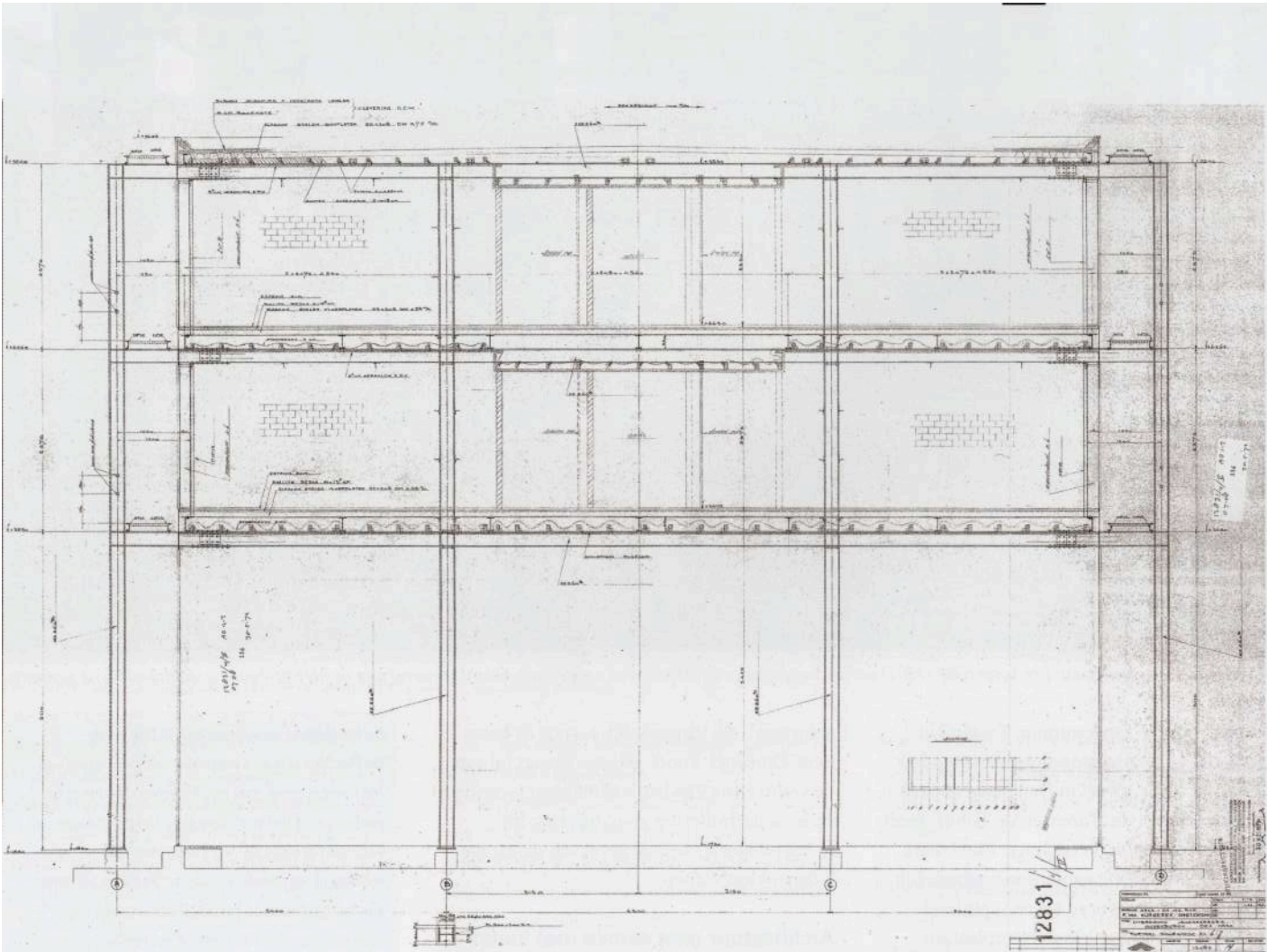
Portaaldoorsnede 6-7 (1971). Vloerbouw: 3 cm Estrich, Hollith beton 4-13,5 cm, Elascor vloerplaten 95x208 (0,88 mm dik), 2 cm 'steendeken', 3,5 cm Heraklin EPV.
