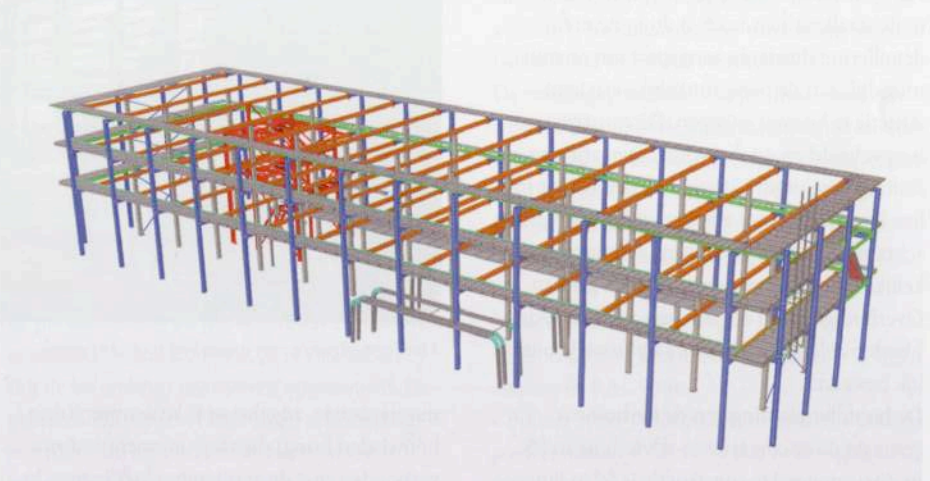
Gehele staalconstructie.
