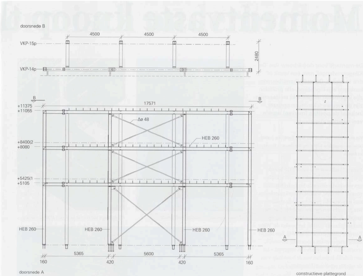
Doorsnede kopgevel (2023). Kanaalplaatvloeren met constructieve druklaag.
